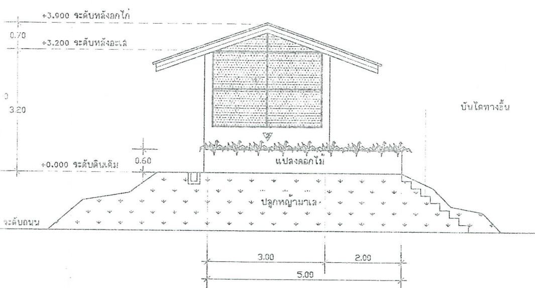
รูปด้านข้าง 1 : 100
